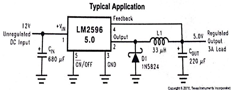
Fig: 3.16: DC-DC Buck Converter
